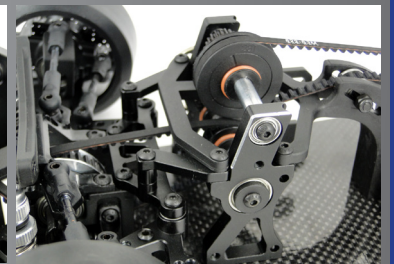
EVOL 用 アルミ製ローターハブ DL170 ¥2,400-(税抜き) ※リア用 左右2個入り※
