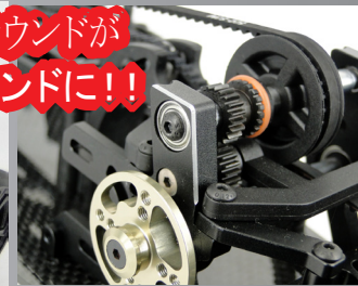
EVOL 用 アルミ製スパーホルダー DL186 ¥1,950-(税抜き)
